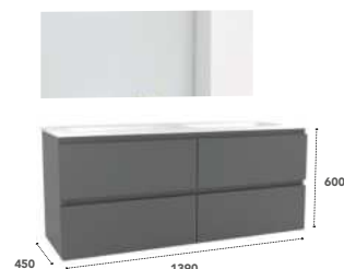
1400 mm (Double vasque)
