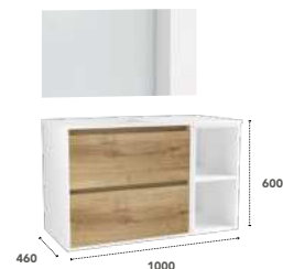
1000 mm avec niches
